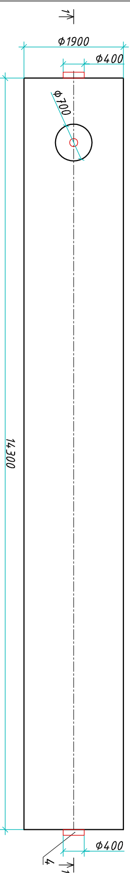
Вид сверху
